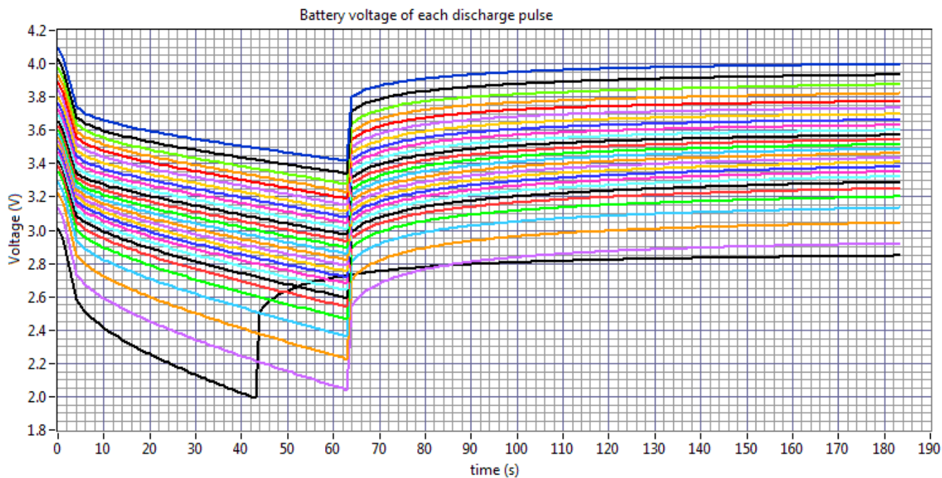
Obrázek 2.14: Zkouška pulzního vybíjení: průběh napětí všech 27 vybíjecích pulzů a následný průběh zotavení napětí baterie během prvních 3 minut po skončení pulzu. První pulz má pro čas t = 183 s nejvyšší napětí, poslední pulz má pro čas t = 183 s nejnižší napětí.
